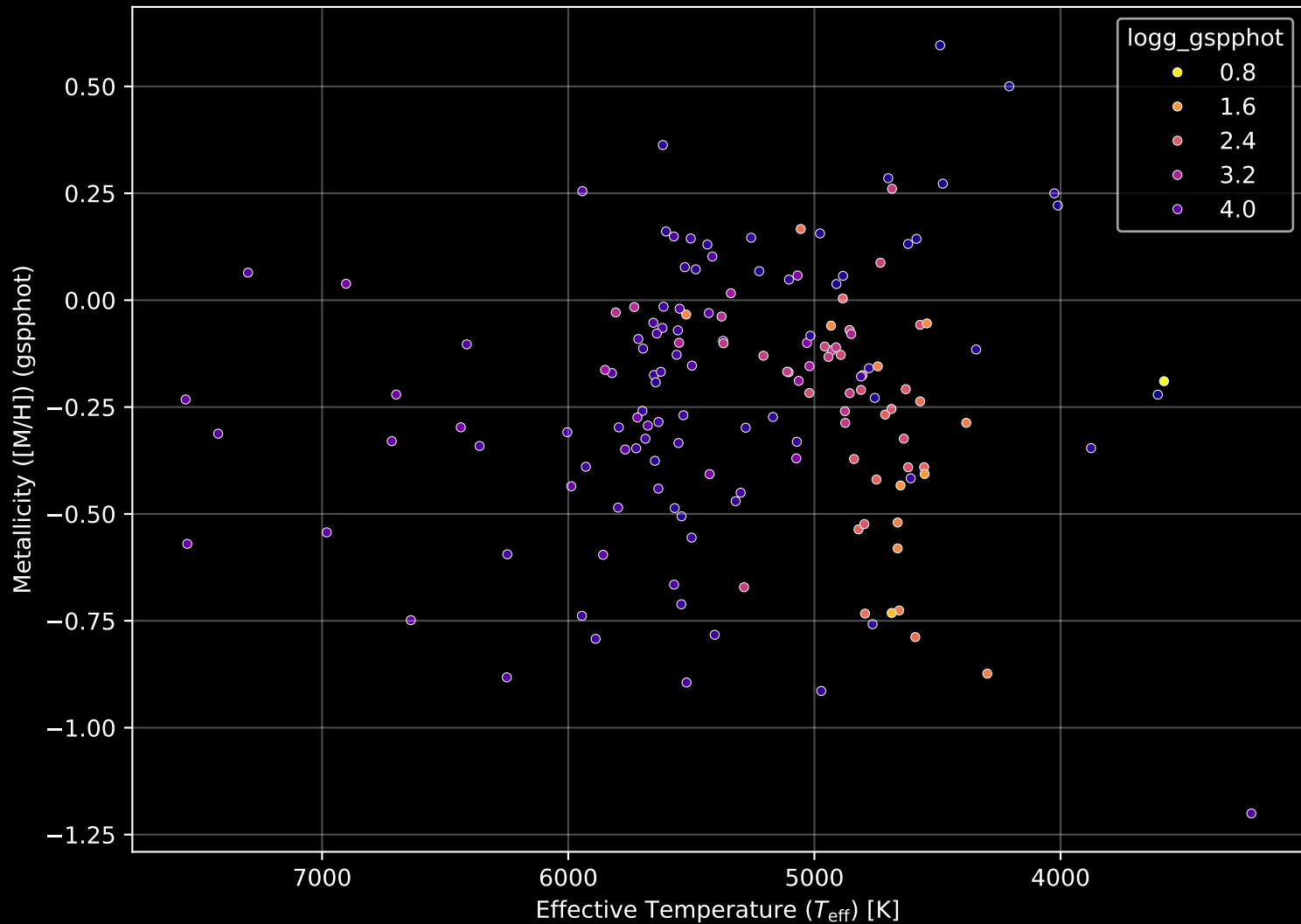
APOGEE DR17 Field: [043+32_MGA] Stellar Population Parameters (n= 156)
